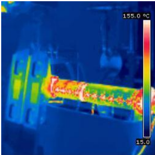
Экструдер без ecoSAVE
